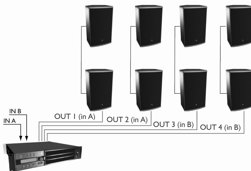
Figure 4 : 8 enceintes 8XT connectées à un contrôleur LA4
