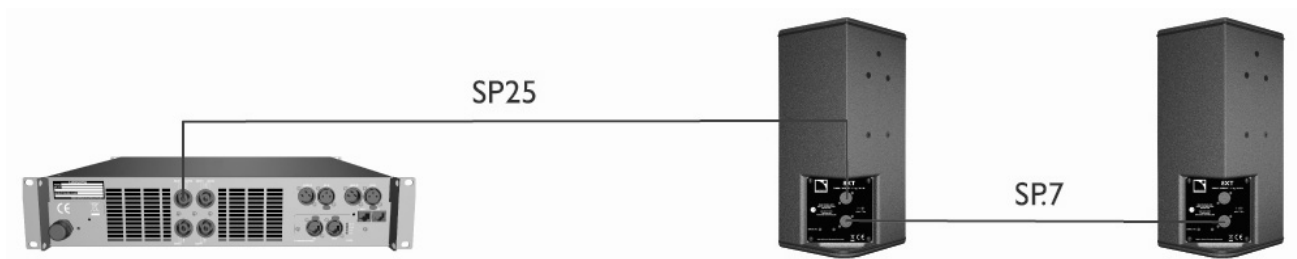
Figure 3 : Raccordement de deux enceintes 8XT en parallèle au contrôleur amplifié LA4
