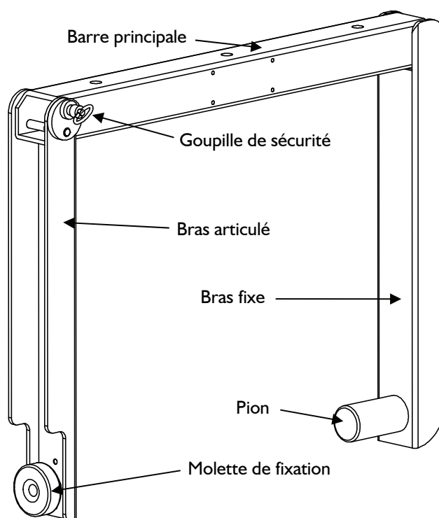
Figure 5 : L'accessoire d'accrochage ETRI5P
