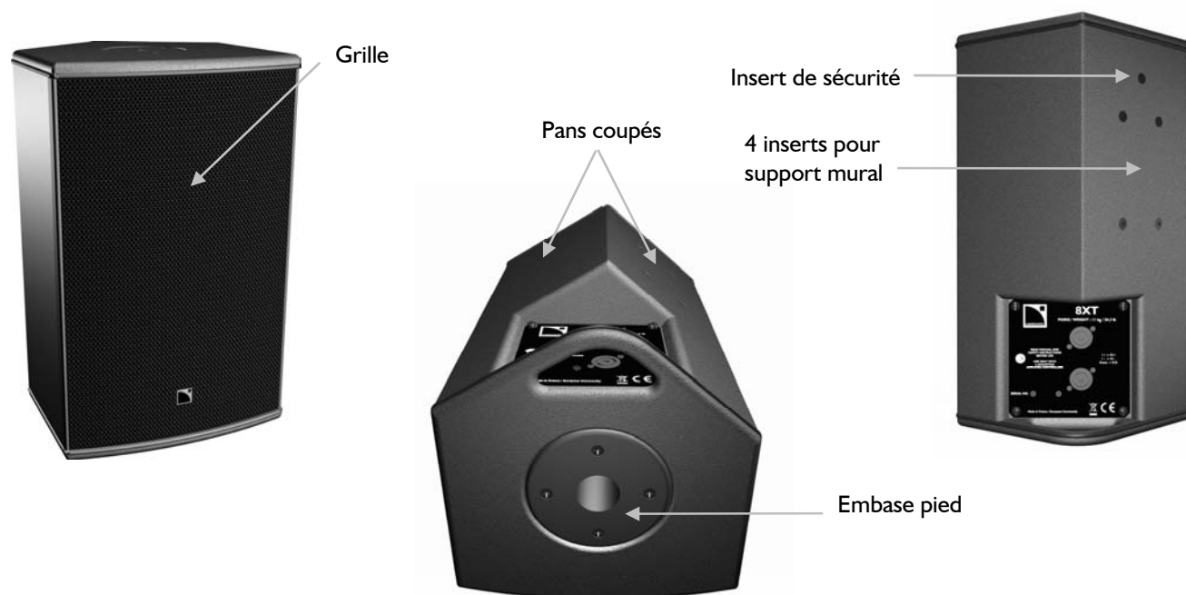
Figure 2 : L'enceinte 8XT et son dispositif d'accrochage
