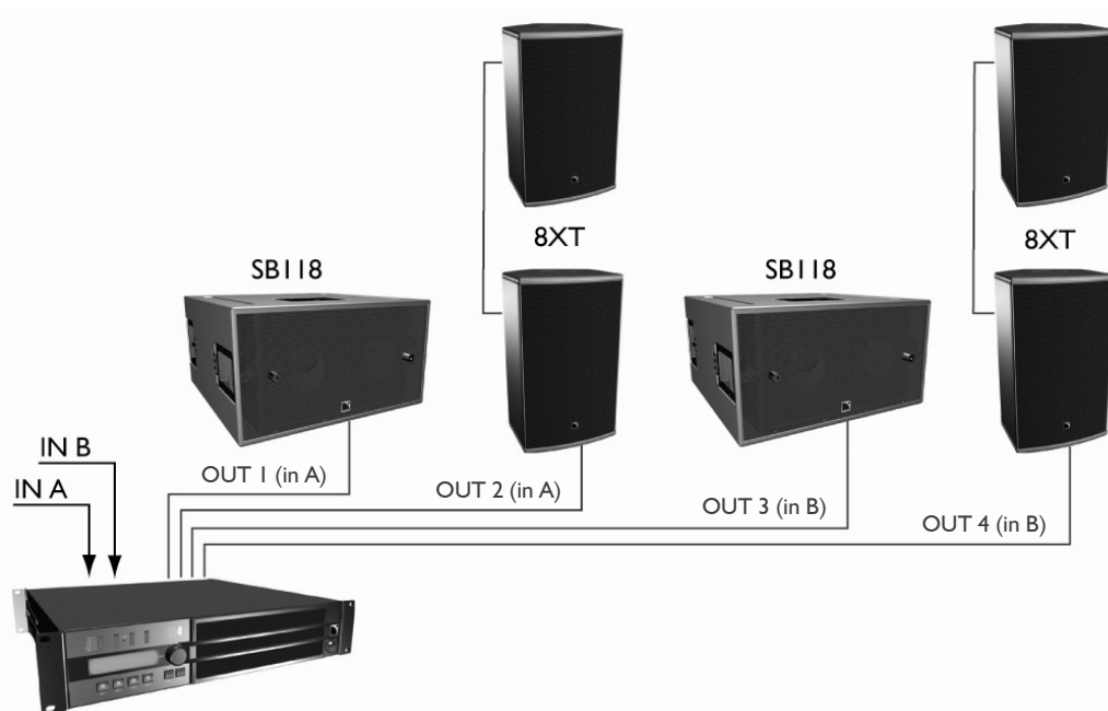
Figure 6 : 2 enceintes sub-graves SBI 18 et 4 enceintes 8XT raccordées au contrôleur amplifié LA4
