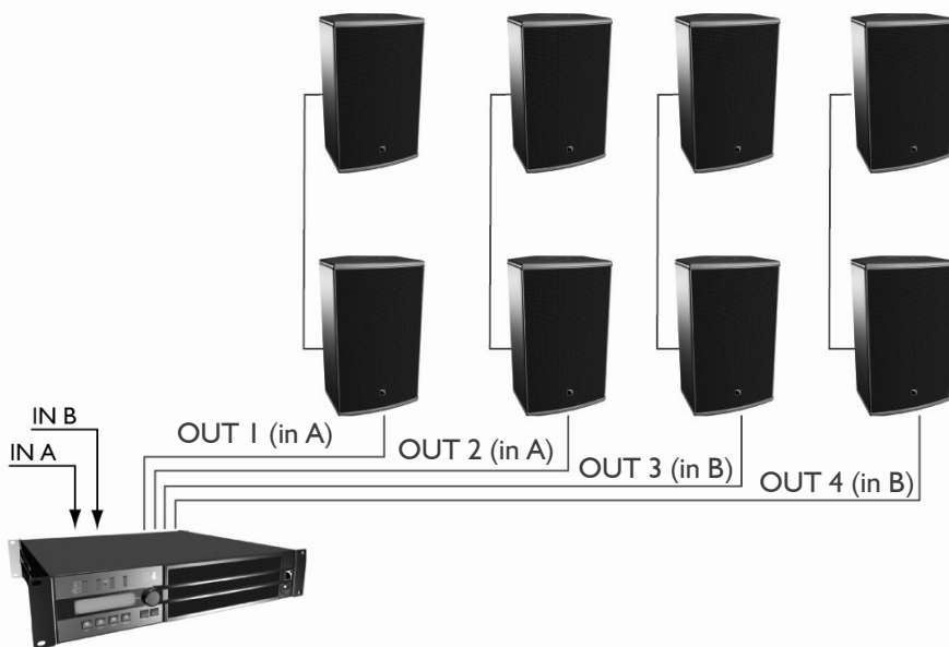
Figure 5 : 8 enceintes 8XT connectées à un contrôleur LA4
