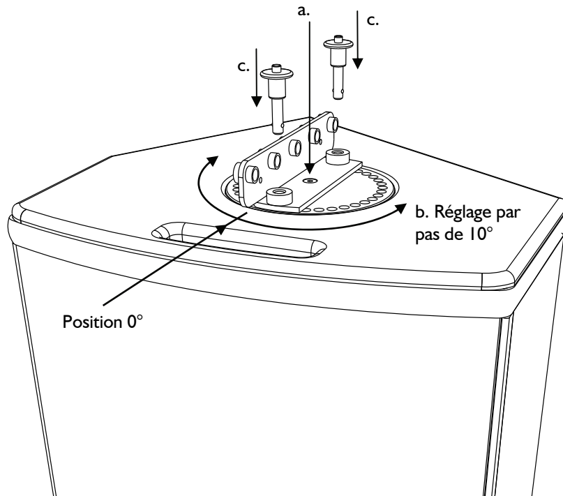
Figure 16 : Positionnement du XTLIFTBAR sur une enceinte pour un réglage en angle de site
